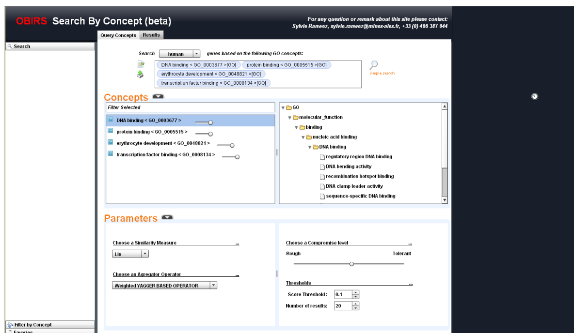
Figure 20 : Interface d'OBIRS permettant d'exprimer une requête
